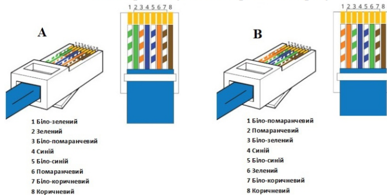
Схема розпинування мережевого дроту
