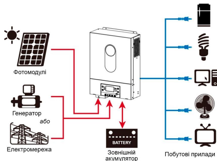
Рисунок 1 Гібридна електростанція
