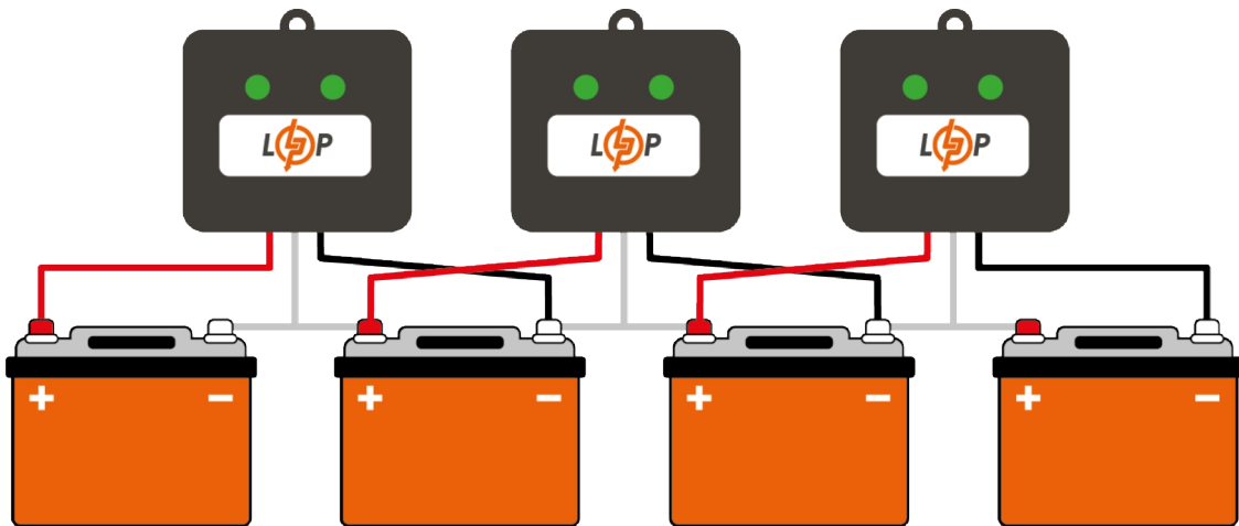
Малюнок 4: 48V акумуляторна збірка
