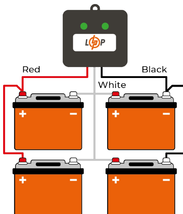
Малюнок 2: 24V акумуляторна збірка з 4-х акумуляторів
