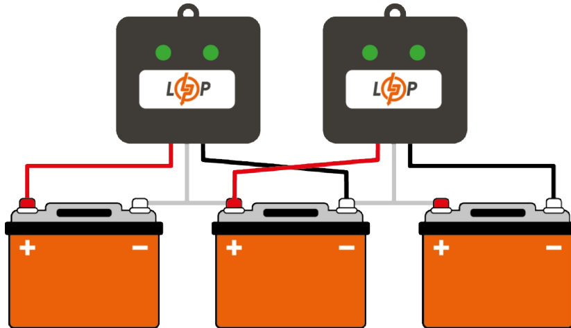
Малюнок 3: 36V акумуляторна збірка
