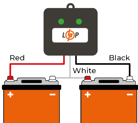
Малюнок 1: 24V акумуляторна збірка з 2-х акумуляторів
