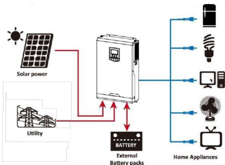
Рисунок 1. Гібридна енергосистема
