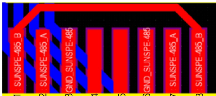
Порт Modbus
