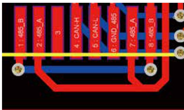
Порт BMS
