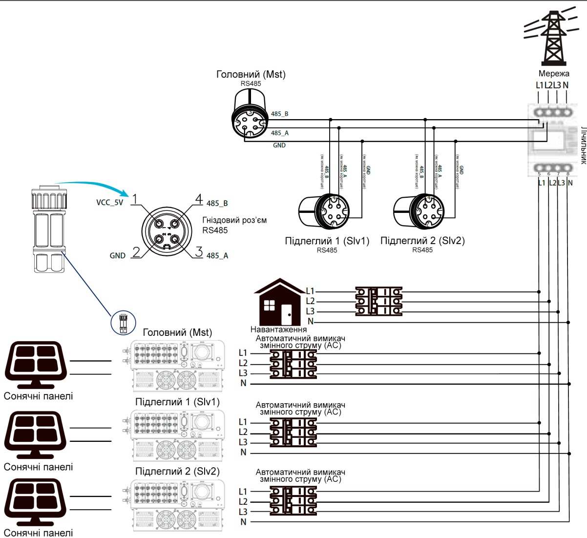
Зображення 7.19 Схема підключення Eastron (Схема наскрізного підключення)
