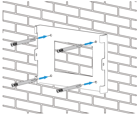
Зображення 4.5 Встановлення монтажної панелі інвертора
