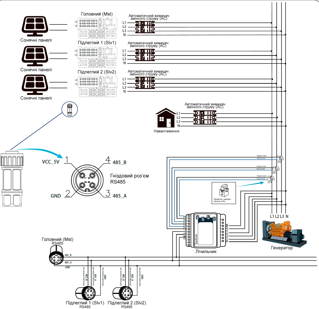
Зображення 7.25 Схема підключення (трифазна мережа)
