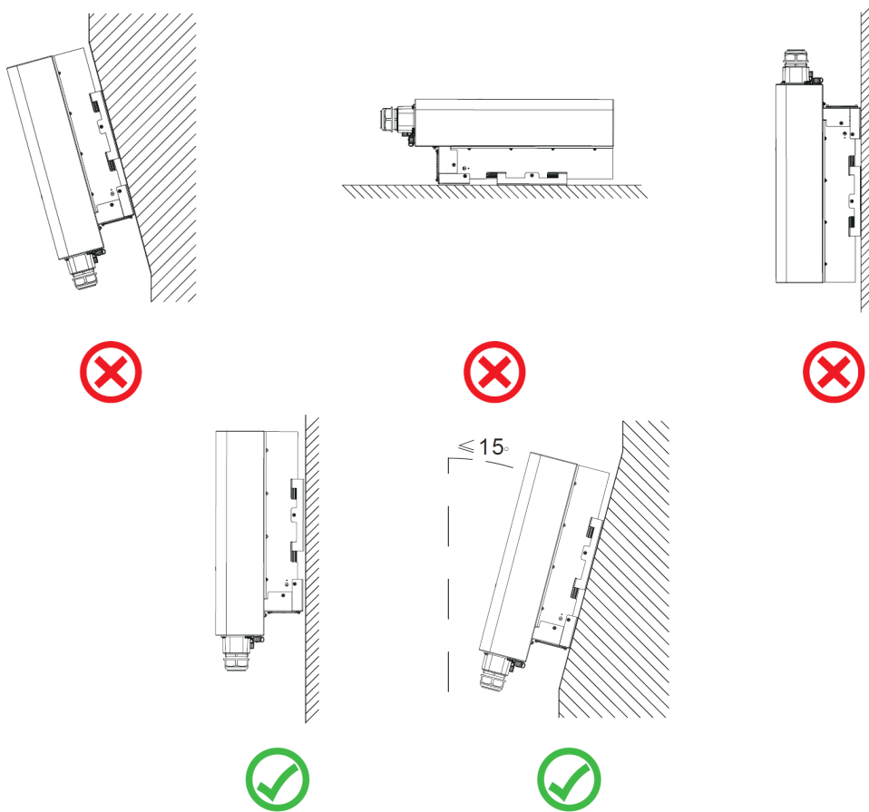
Зображення 4.2 Кут встановлення
