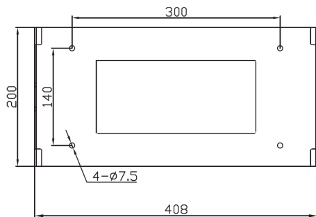
Зображення 4.5 Встановлення монтажної панелі інвертора
