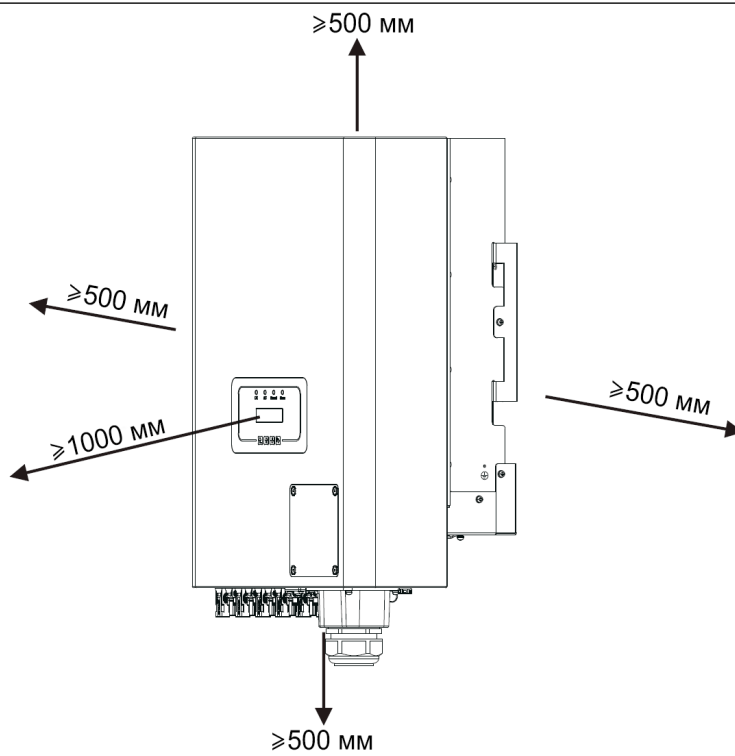
Зображення 4.3 Проміжок при встановленні
