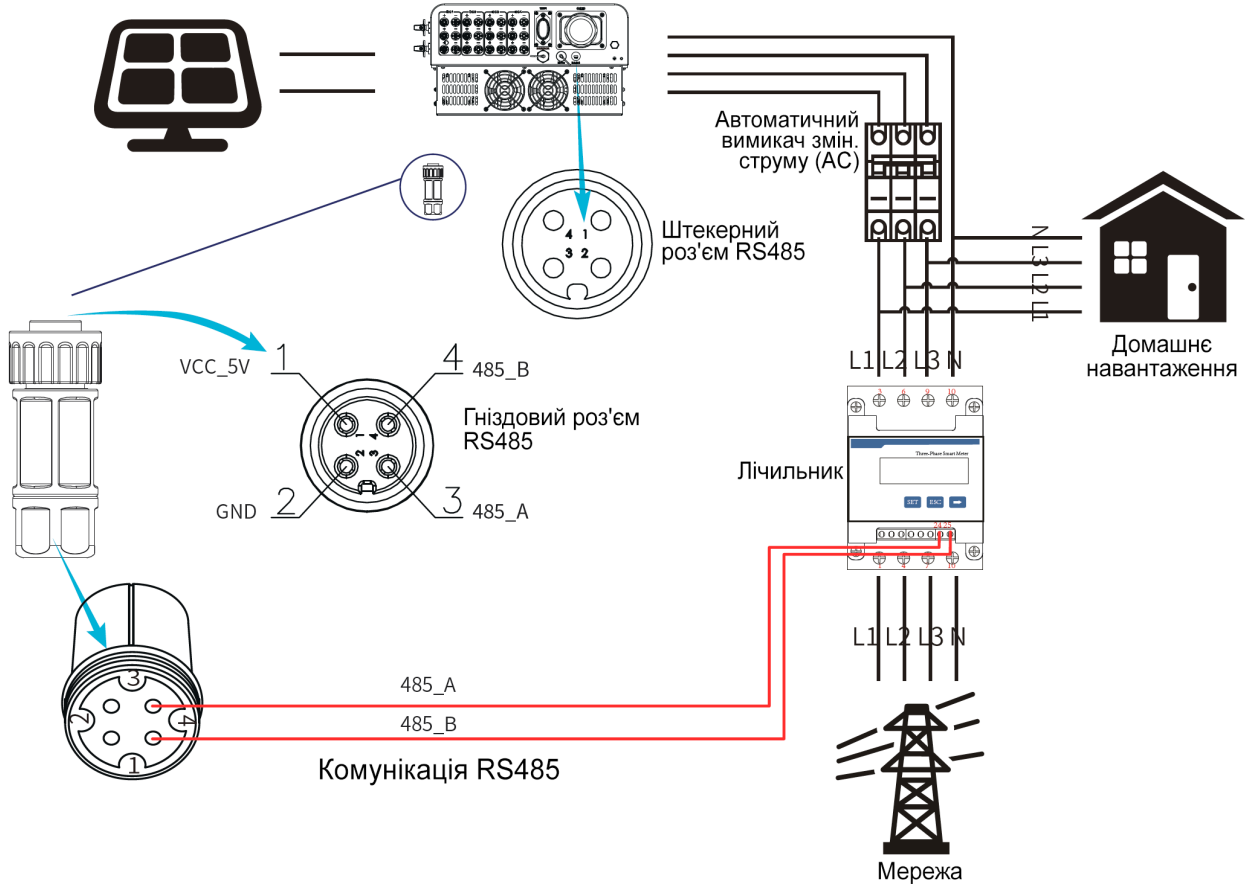
Зображення 7.10 Схема підключення лічильника CHINT
