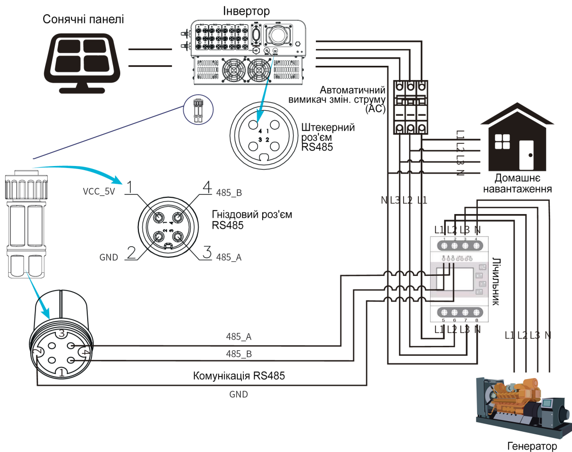
Зображення 7.4 Схема підключення лічильника Eastron
