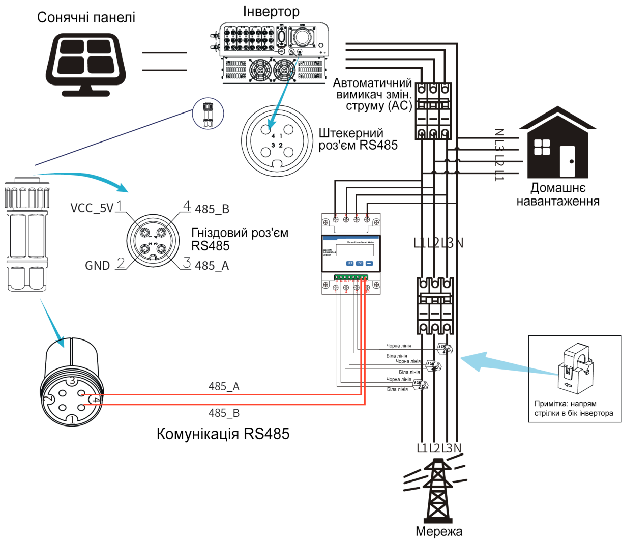
Зображення 7.14 Схема підключення лічильника CHINT
