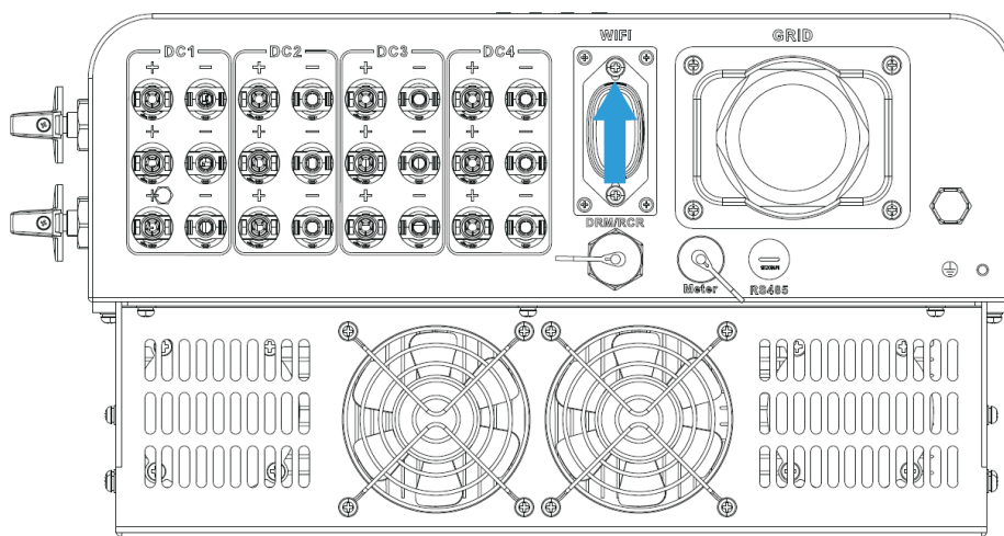
Зображення 5.10 Схема встановлення реєстратора даних
