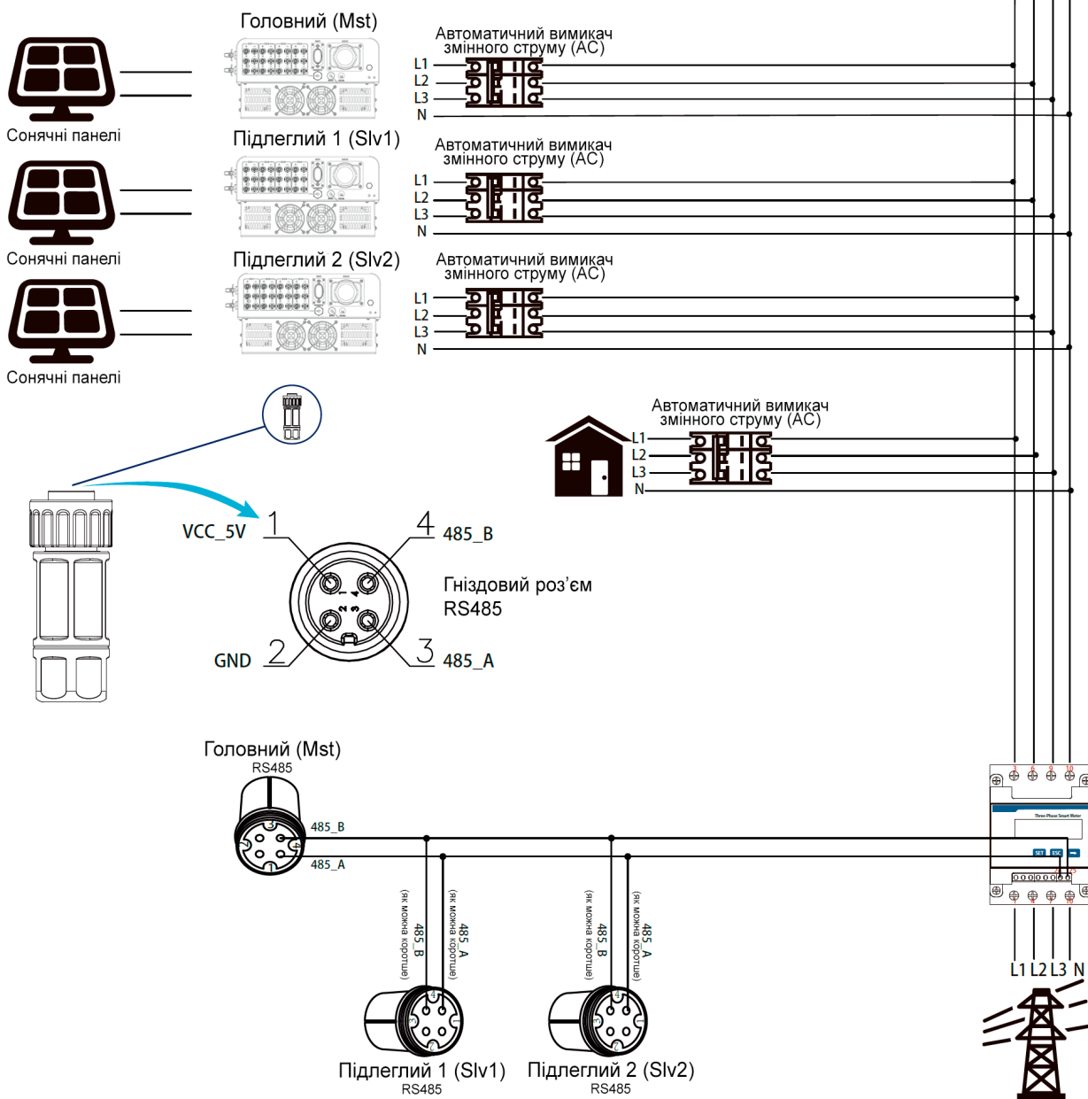
Зображення 7.27 Схема підключення CHINT (Схема наскрізного підключення)
