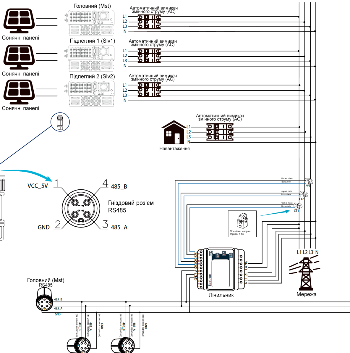
Зображення 7.23 Схеми підключення (трифазна мережа)
