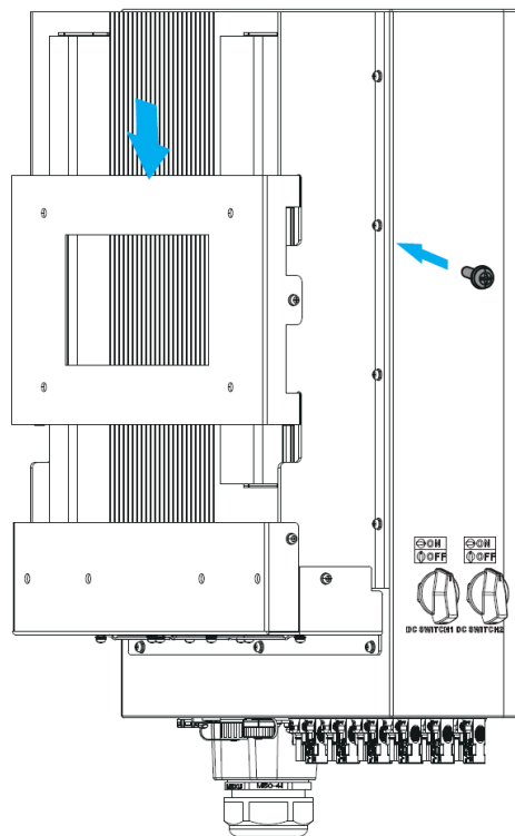
Зображення 4.6 Встановлення інвертора
