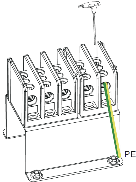
Зображення 5.8 Встановлення заземлювального проводу корпусу
