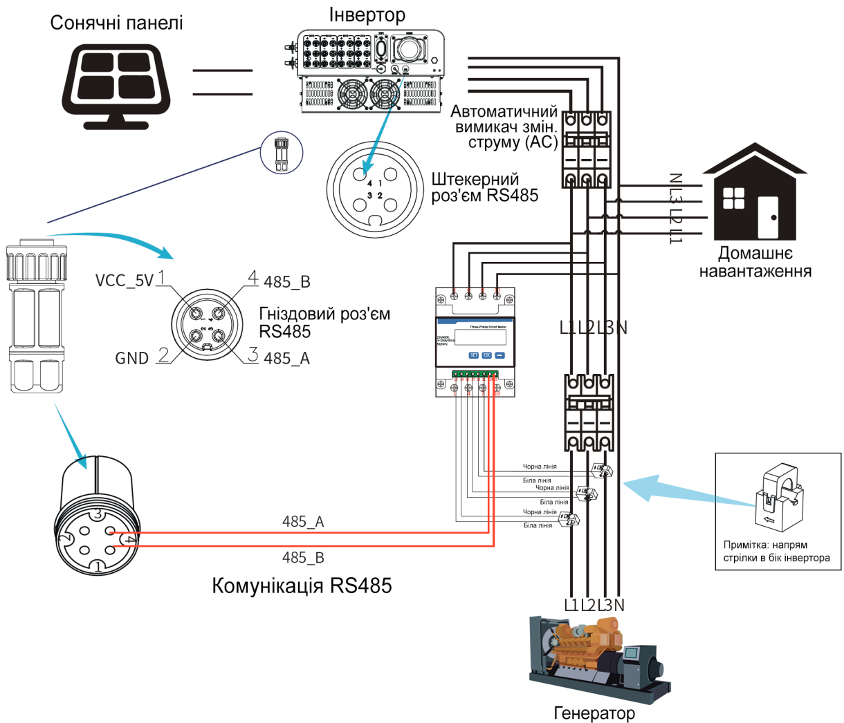
Зображення 7.16 Схема підключення лічильника CHINT
