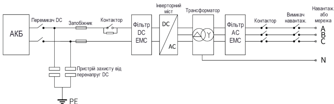
Топологія основної схеми серії PCS для роботи з мережею
